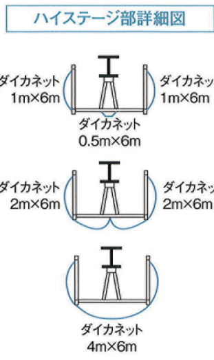
ハイステージ使用時 ハイステージの手すり間や足場板の隙間からの墜転落を防止します。
